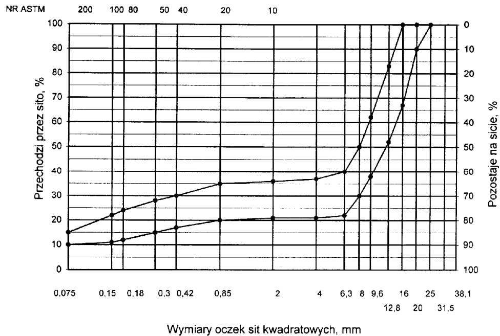
Rys. 5. Krzywe graniczne uziarnienia mieszanki mineralnej BA od 0 do 20 mm (mieszanka o nieci ąglým uziarnieniu) do warstwy ścieralnej nawierzchni drogi o obciążeniu ruchem od KR3 do KR6
